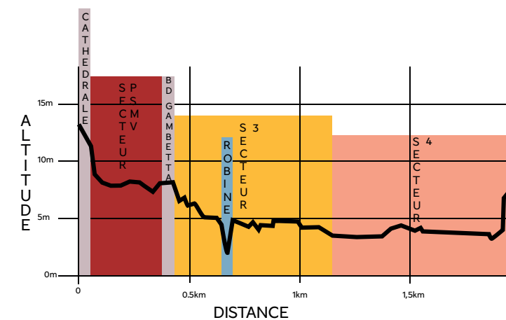
coupe de principe sur le secteur
