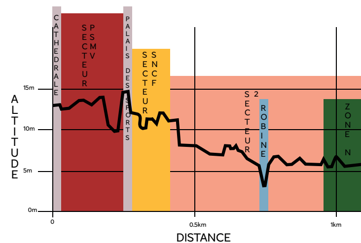
coupe de principe sur le secteur
