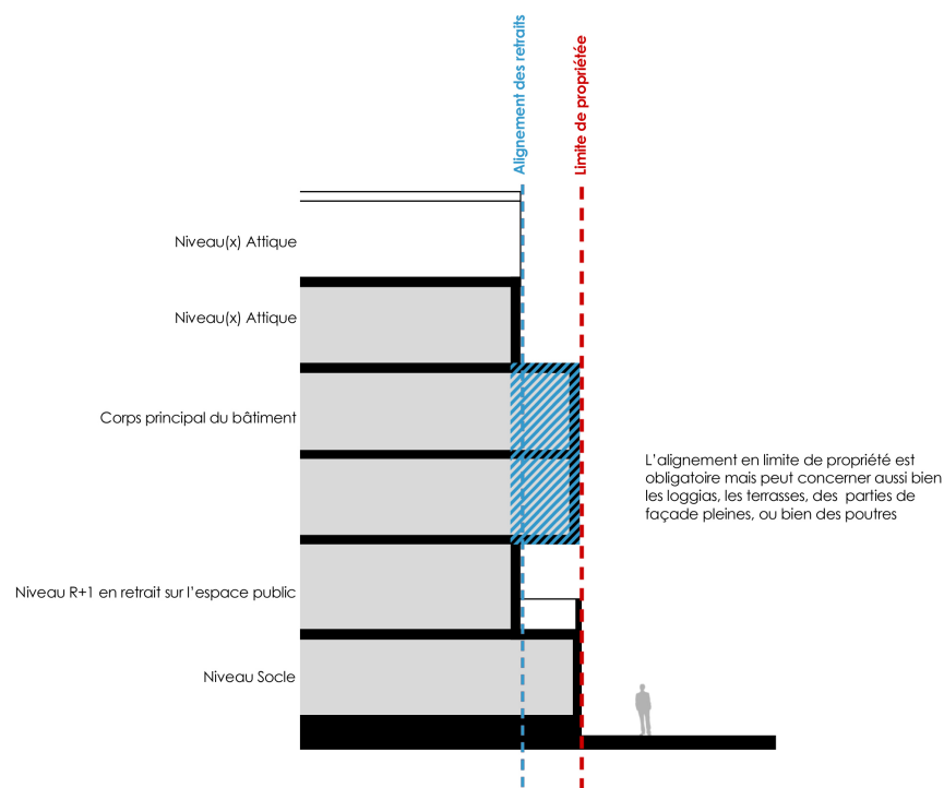
Principe général de superposition des strates bâties sur espace public
